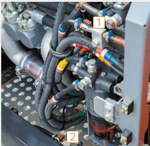
① 燃料コック ② 燃料ドレンコック
