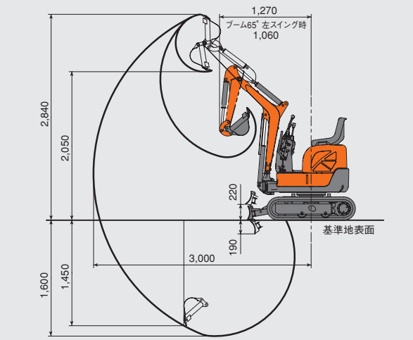
■作業範囲図
