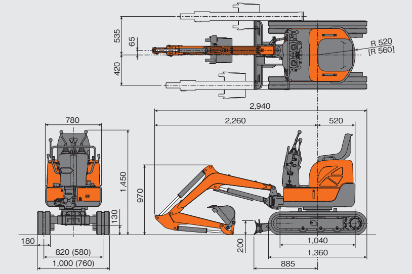
■寸法図
