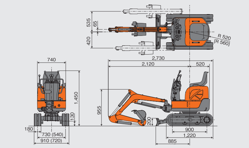
■寸法図
