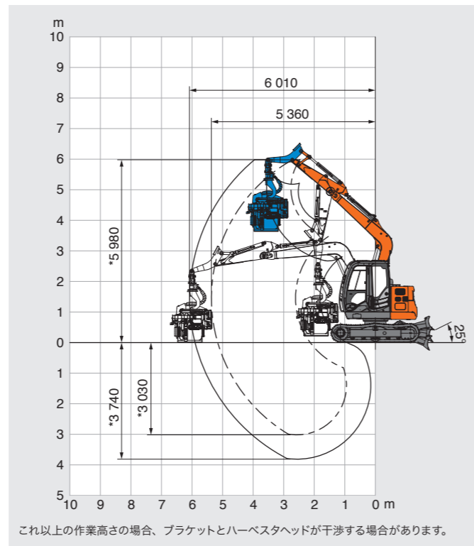
● ZX75USL-5B ハーベスタパッケージ
