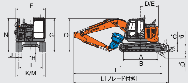
● ZX135US-6 グラップルパッケージ
