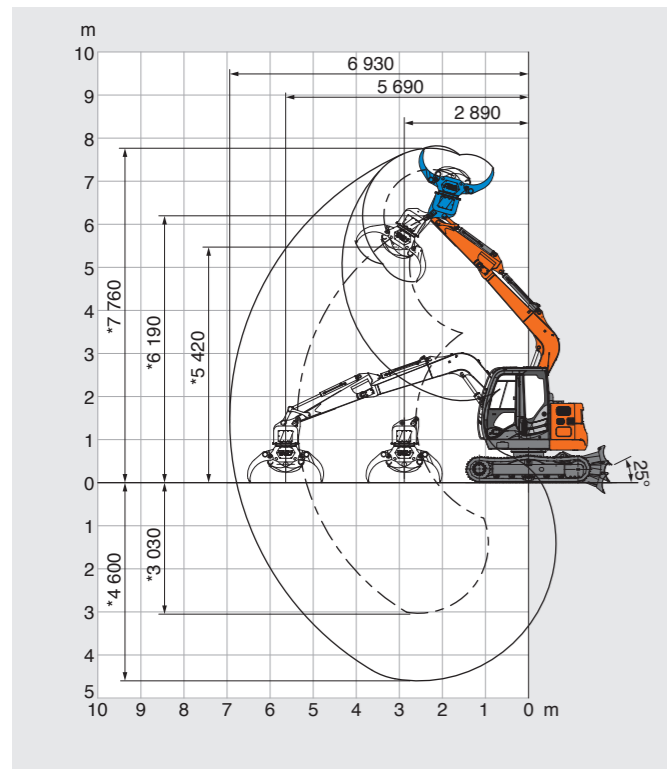
● ZX75US-5B グラップルパッケージ
