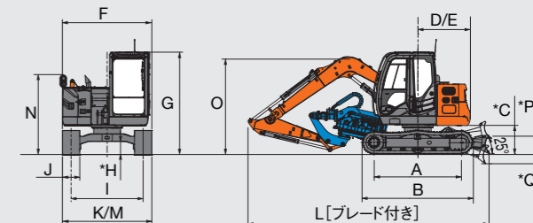
● ZX75USL-5B ハーベスタパッケージ
