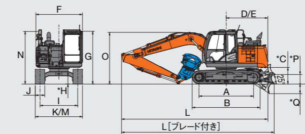
● ZX120-6 グラップルパッケージ
