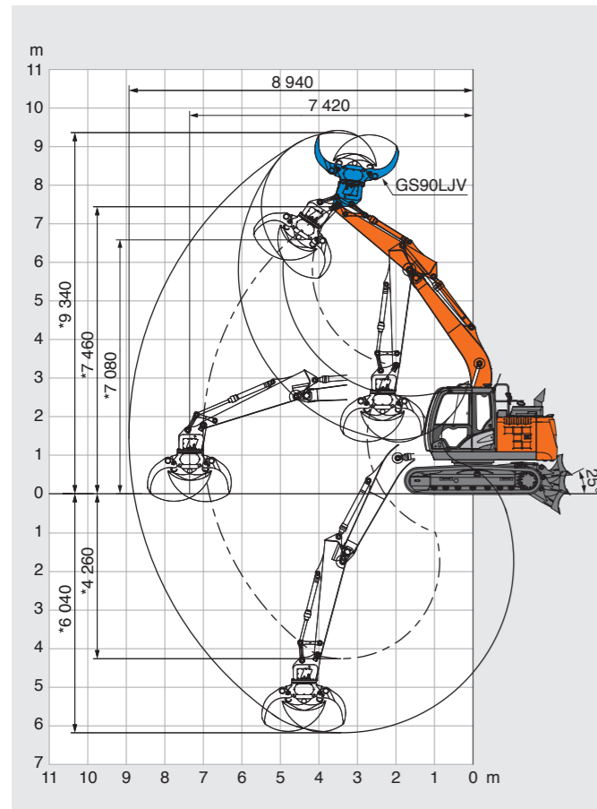
● ZX120-6 グラップルパッケージ
