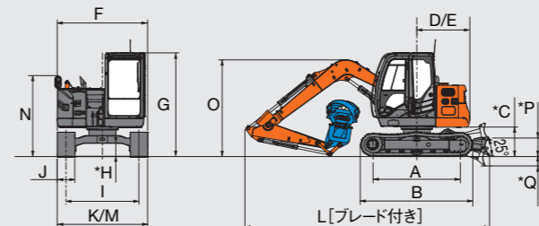
● ZX75US-5B グラップルパッケージ
