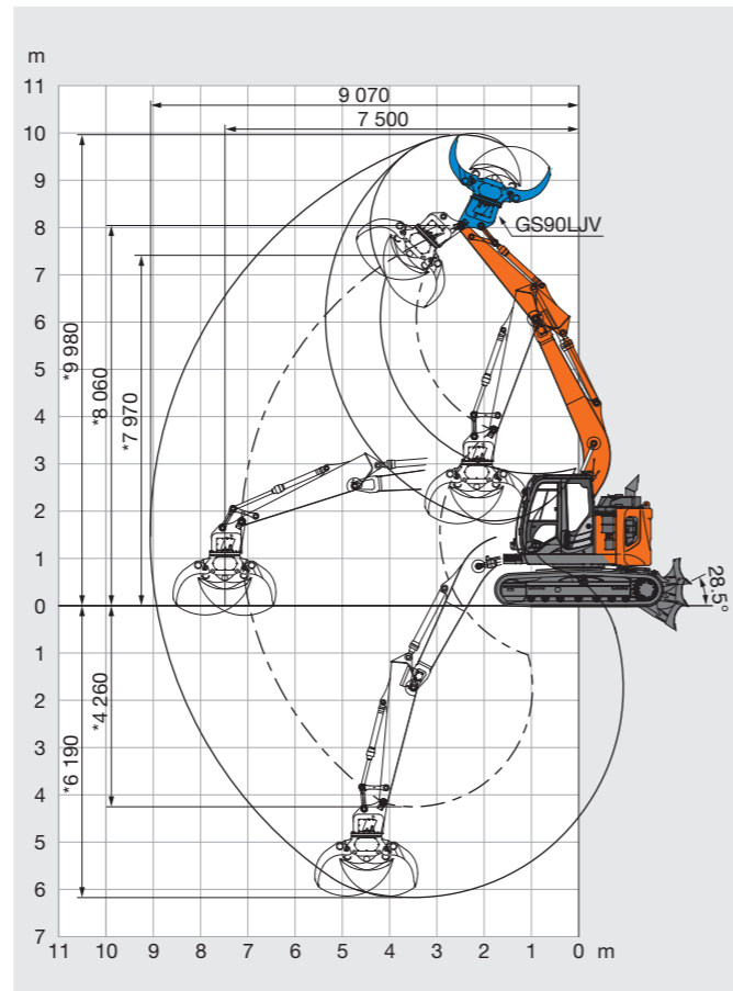
● ZX135US-6 グラップルパッケージ
