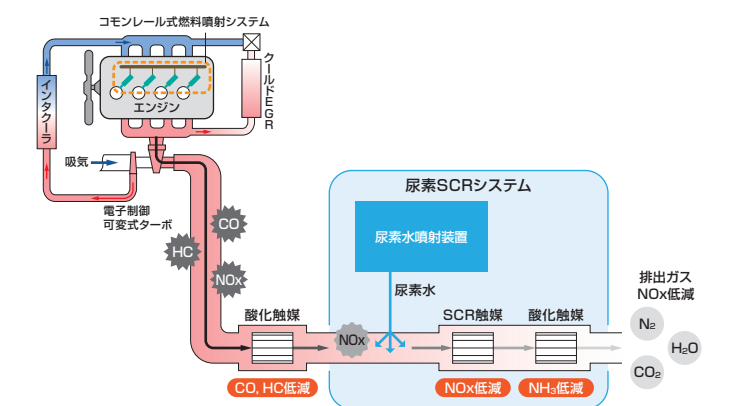
エンジンシステム図
